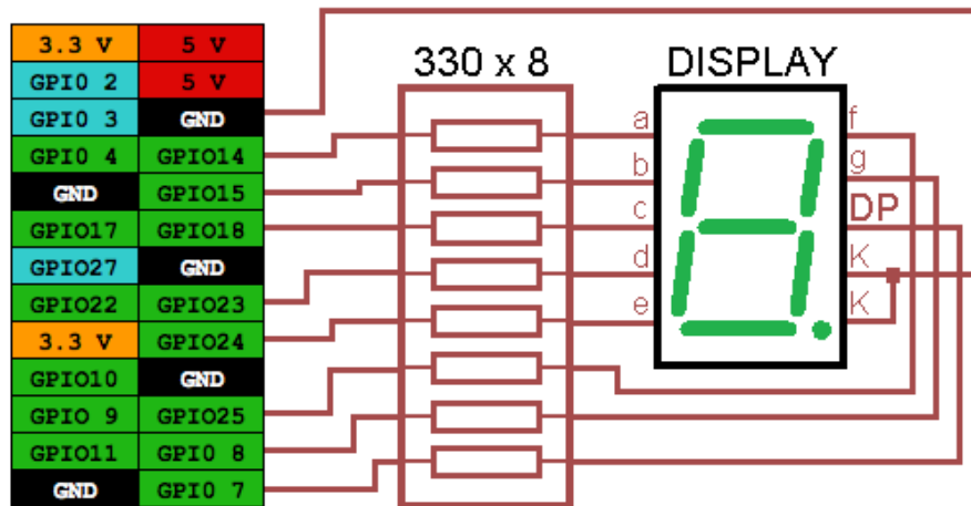
Esquema electrónico del montaje propuesto.
